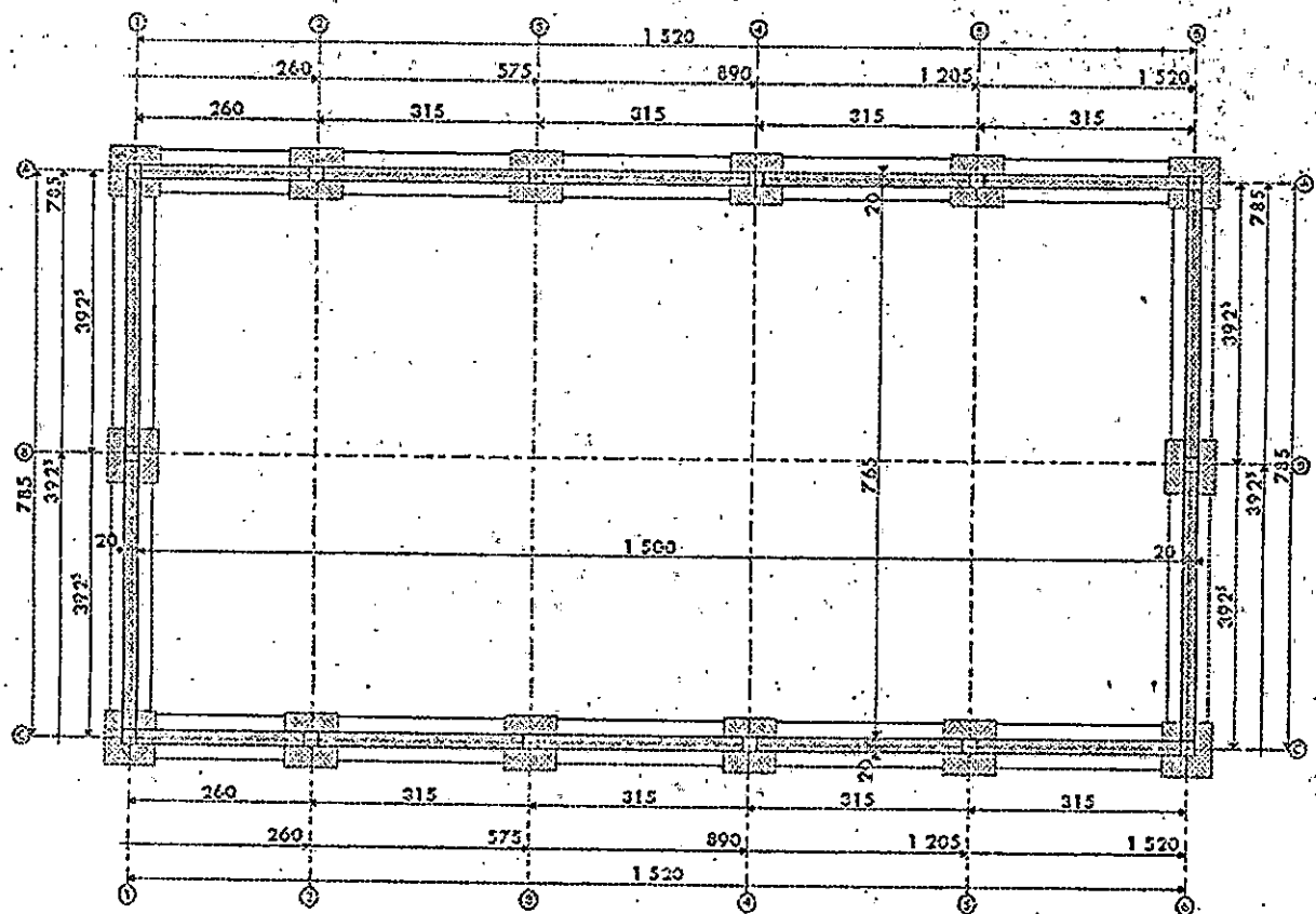
PLAN DE FONDATION - FOUNDATION PLAN
