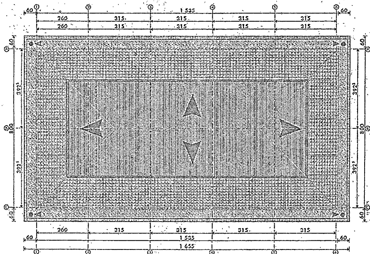
PLAN DE TOITURE - ROOF PLAN
